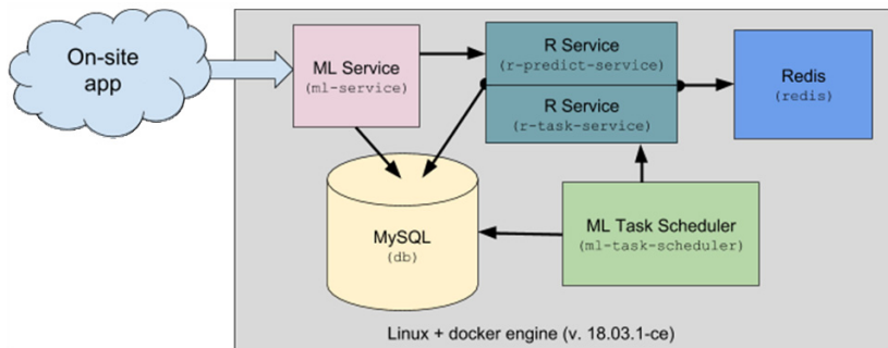
Рис. 619 — Компоненты сервиса машинного обучения
