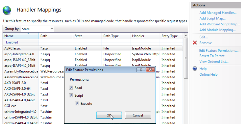
Рис. 605 — Проверка необходимых параметров в окне [Edit Feature Permissions]
